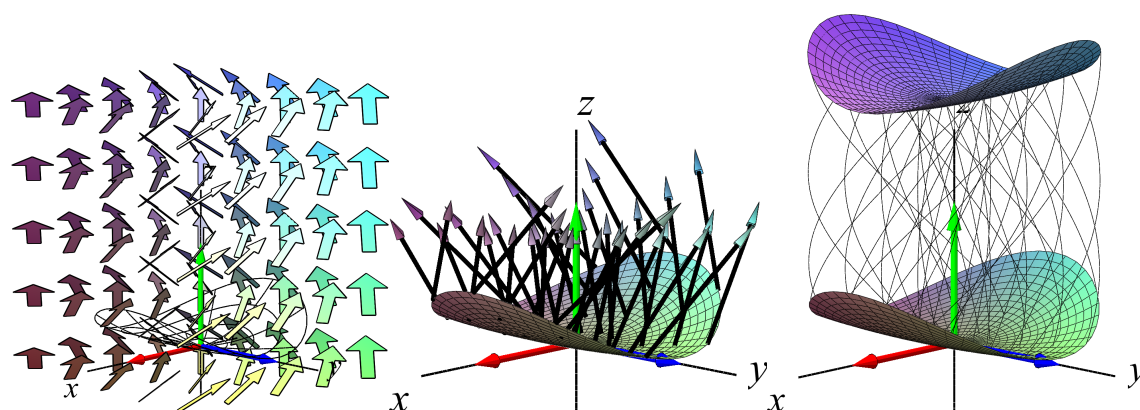
Figure 28.7: Et roterende vektorfelt, og tilsvarende kort-tids flow af en elliptisk paraboloid. I forhold til cirkelskivenormalen er fluxen og volumen-tilvæksten positiv. Se eksempel 28.9.
