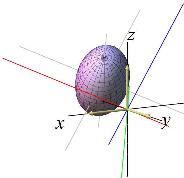
Figure 22.6: Niveaufladen \mathcal{K}_0(f) for den funktion som er analyseret i eksempel 22.5. Det nye roterede koordinatsystem hvori ellipsoiden har reduceret form er antydet med den røde \tilde{x} -akse, bl \tilde{y} -akse, og grønne \tilde{z} -akse.
